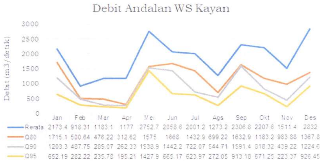
Gambar 5.4 Debit Andalan Q80,Q90 dan Q95 WS Kayan
