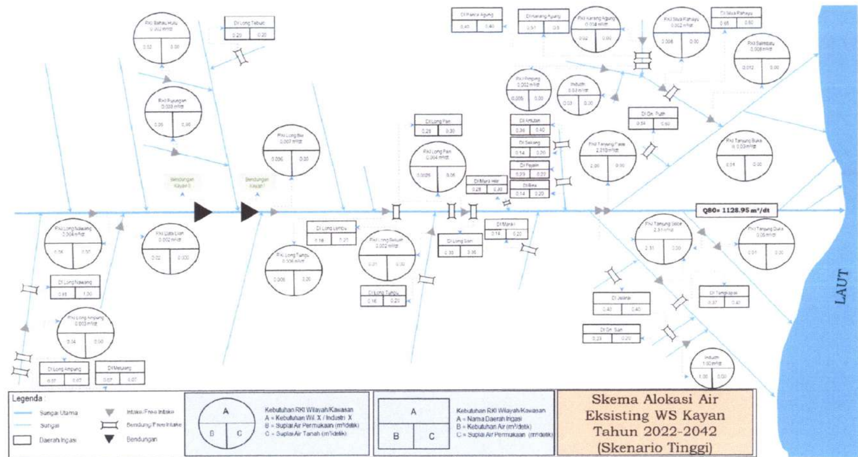
Gambar 5.10 Skema Alokasi Air Skenario Tinggi WS Kayan 2022-2042
