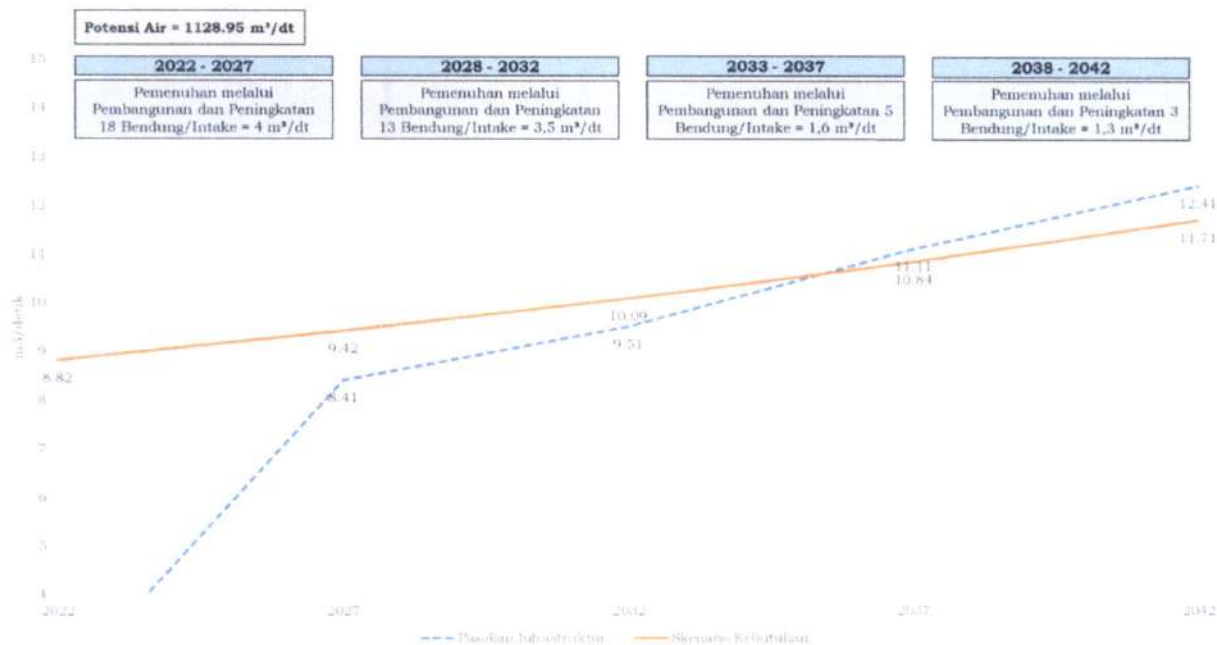
Gambar 5.6. Neraca Air WS Kayan Skenario Sedang
