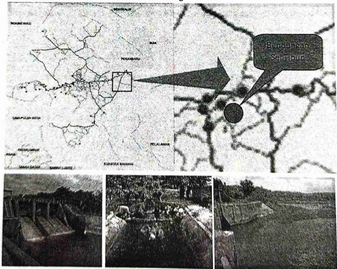
Gambar 4.68. Kondisi dan Letak Bendungan Sei Tibun
