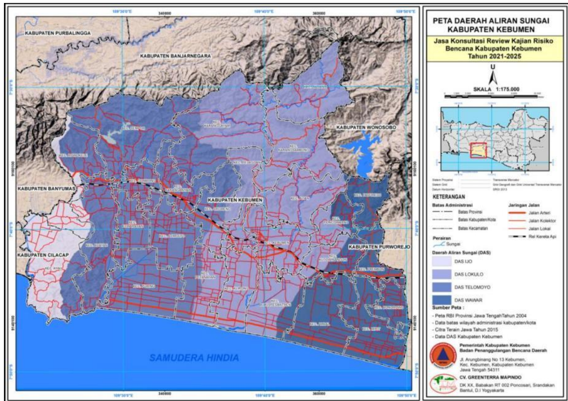
Gambar 2.1. Peta Daerah Aliran Sungai Kabupaten Kebumen
