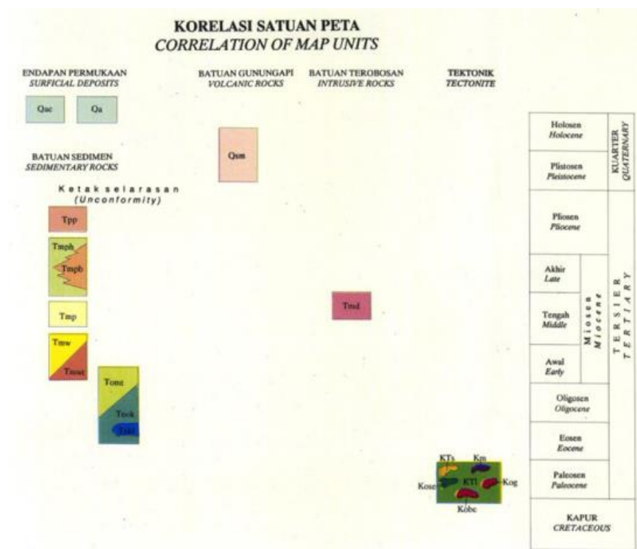
Gambar 2.3. Struktur Geologi Kabupaten Kebumen
