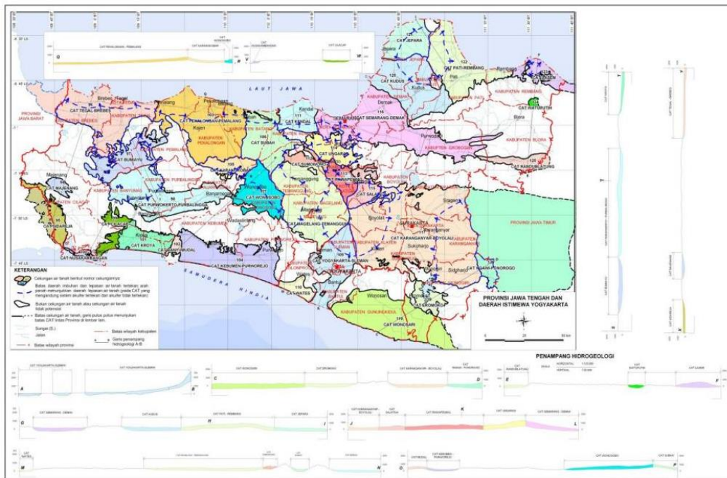
Gambar 2.2. Peta Hidrogeologi Provinsi Jawa Tengah dan Daerah Istimewa Yogyakarta
