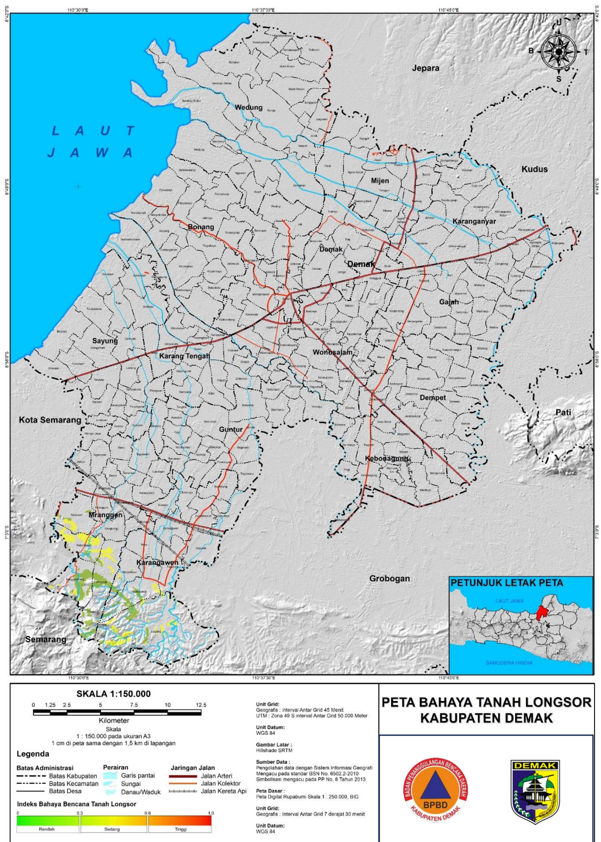
Gambar 3. 118 Peta Bahaya Bencana Tanah Longsor Demak
