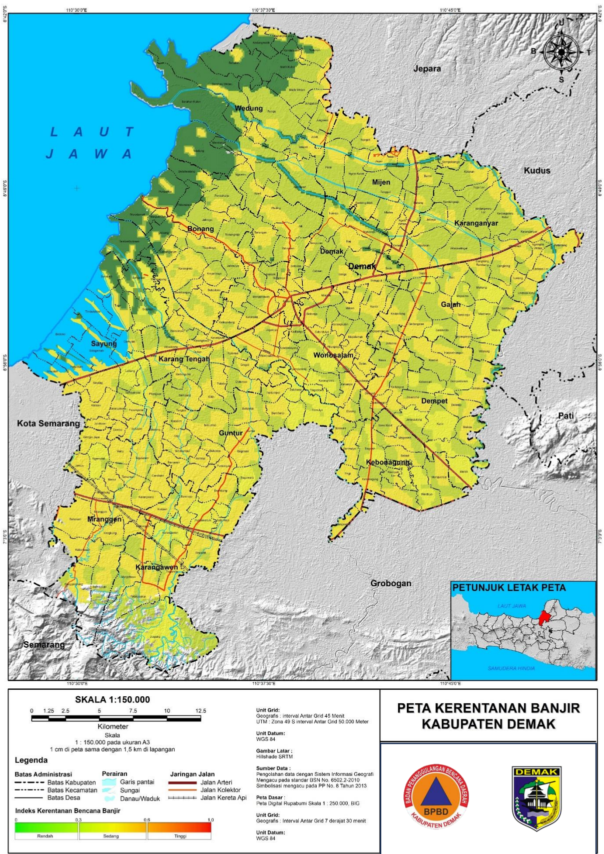
Gambar 3. 119 Peta Kerentanan Bencana Banjir Kabupaten Demak
