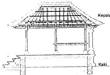
STRUKTUR MASIF DAN RANGKA
