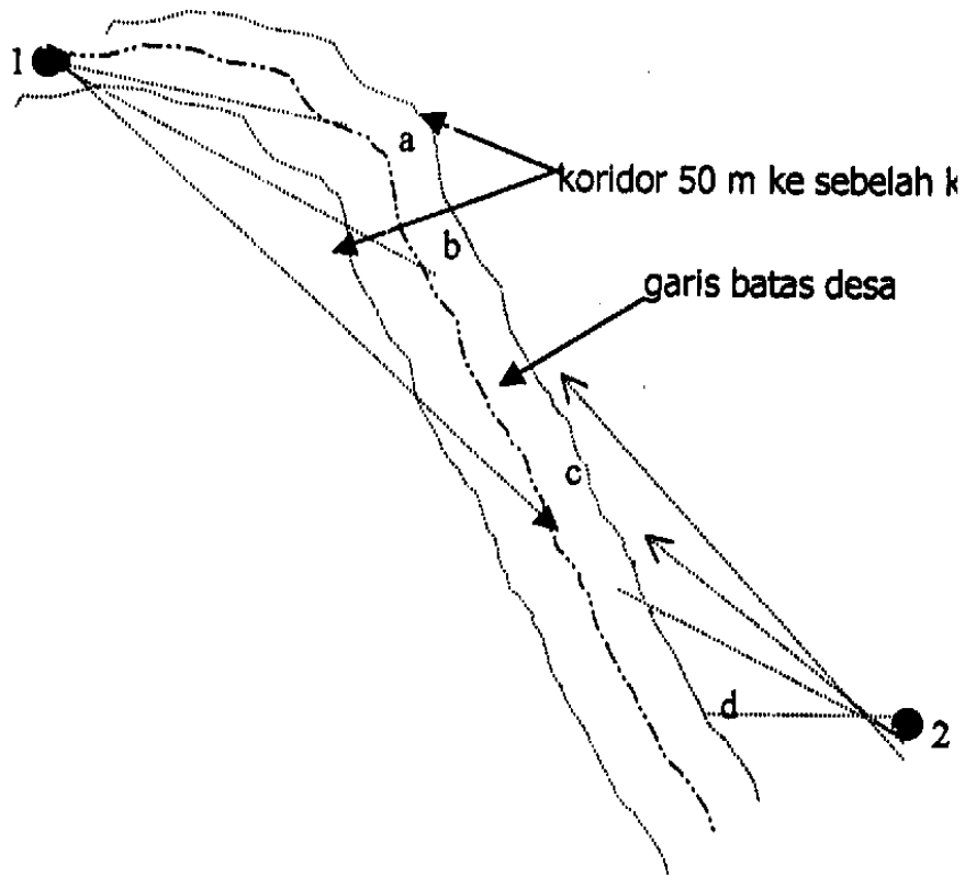
Gambar 16 Pengukuran tachimetri sepanjang garis batas
