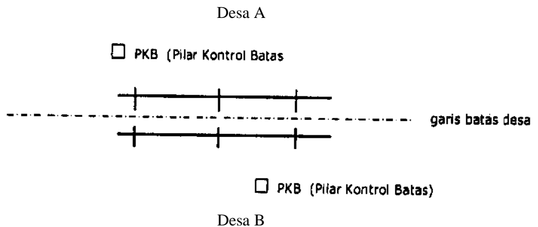
Gambar 6 Jalan Kereta Api Sebagai Batas Desa
