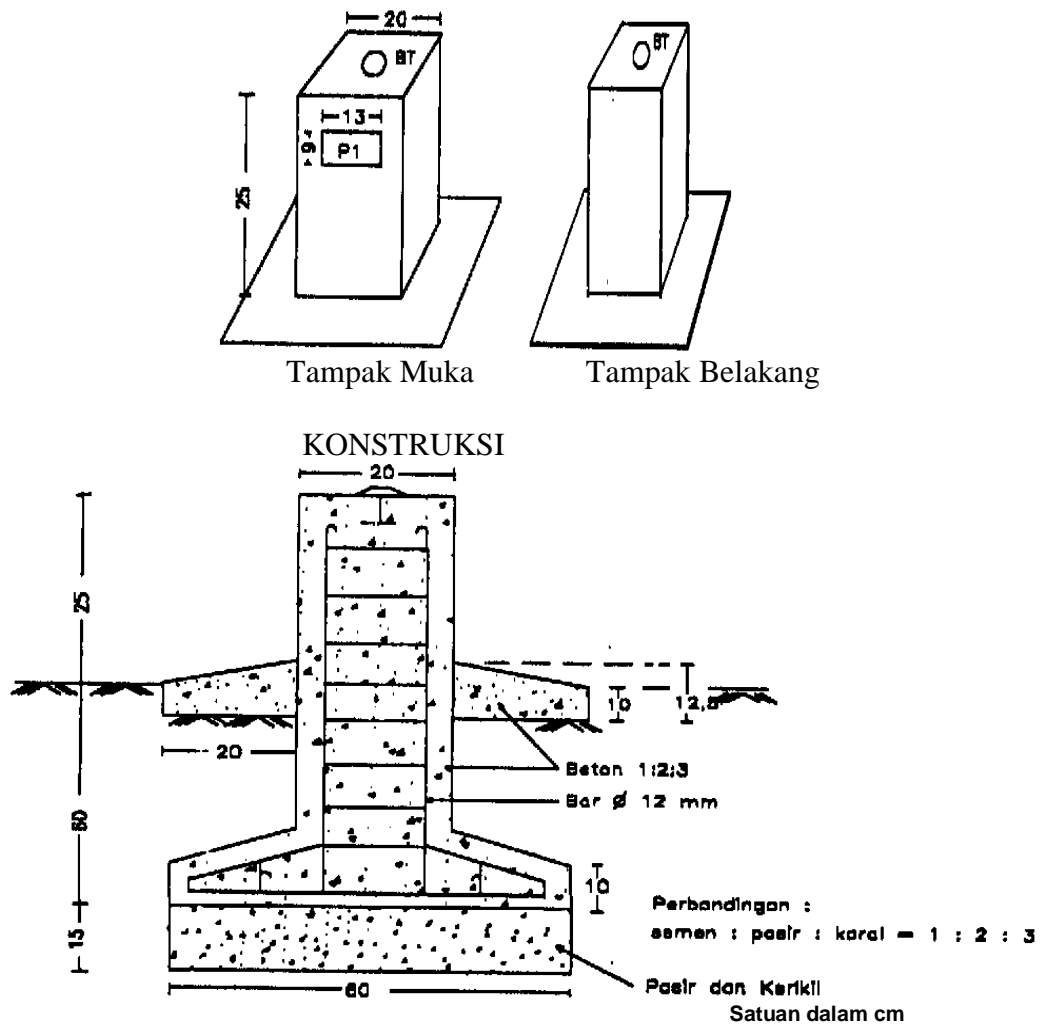
(a) Konstruksi Pilar Gambar 8 Pilar Tipe D - Batas desa
