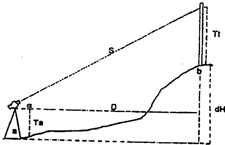
Gambar 17. Pengukuran Tachimetri
