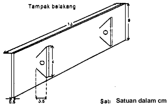
Gambar 10. Plak, terbuat dari kuningan
