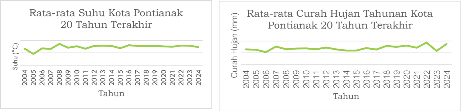
Grafik 2.1 Perubahan Rata-Rata Curah Hujan dan Suhu Udara
