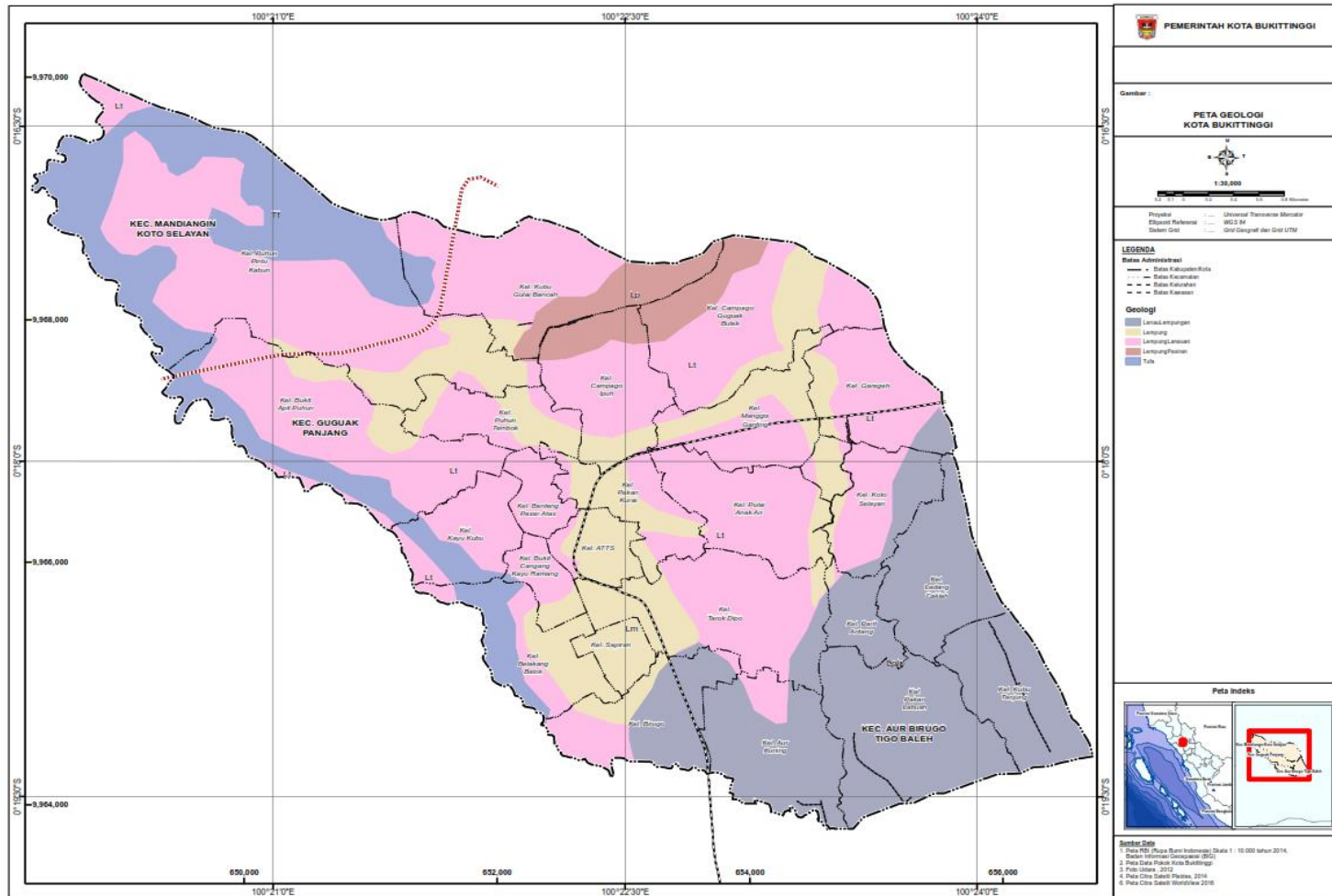
Gambar 2.3. Peta Geologi Kota Bukittinggi
