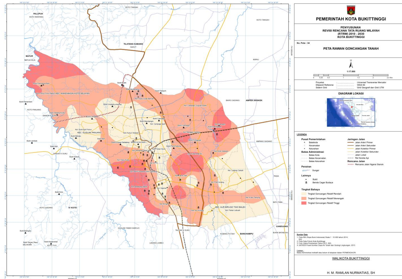
Gambar 2.6. Peta Guncangan Tanah Kota Bukittinggi
