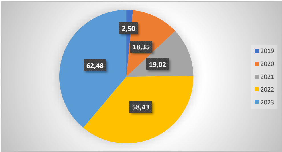
Gambar 2.41 Persentase Peningkatan Konstruksi Jalan Kabupaten Tahun 2019-2023
