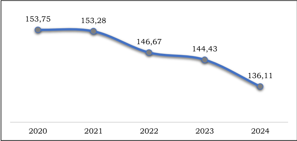
Gambar 2.14. Indeks Risiko Bencana Provinsi Kalimantan Timur Tahun 2020-2024 (Sumber: BPBD Provinsi KALTIM, 2025)
