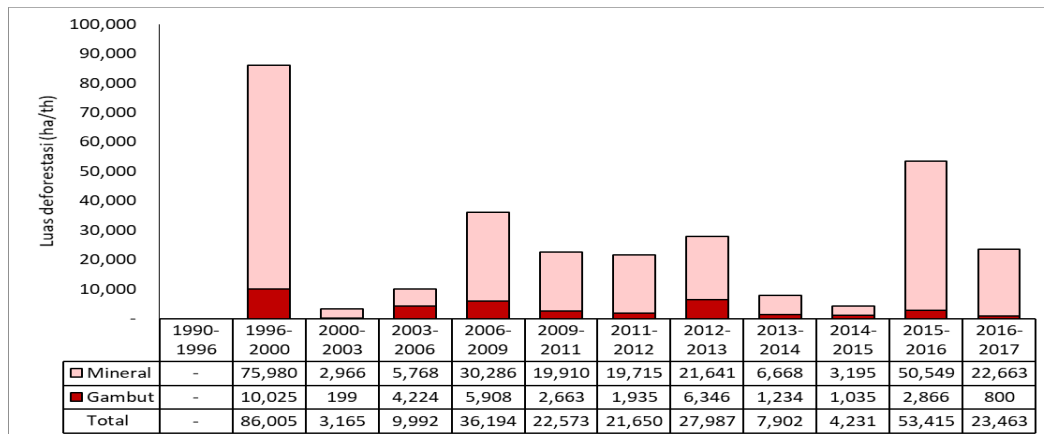
Gambar 2.62. Luas deforestasi di Aceh pada periode 1990–2017
