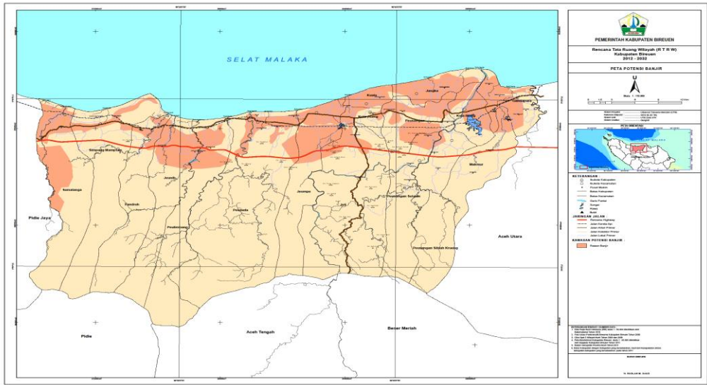
Sumber : Bappeda Kabupaten Bireuen, 2019 Gambar 2.2 Peta Potensi Banjir Kabupaten Bireuen
